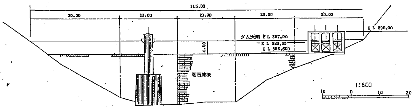
ダム越流部標準断面図
