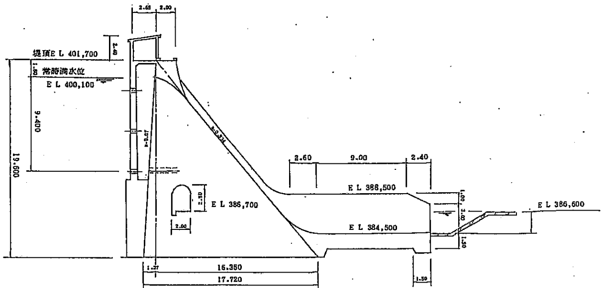
ダム越流部標準断面図
