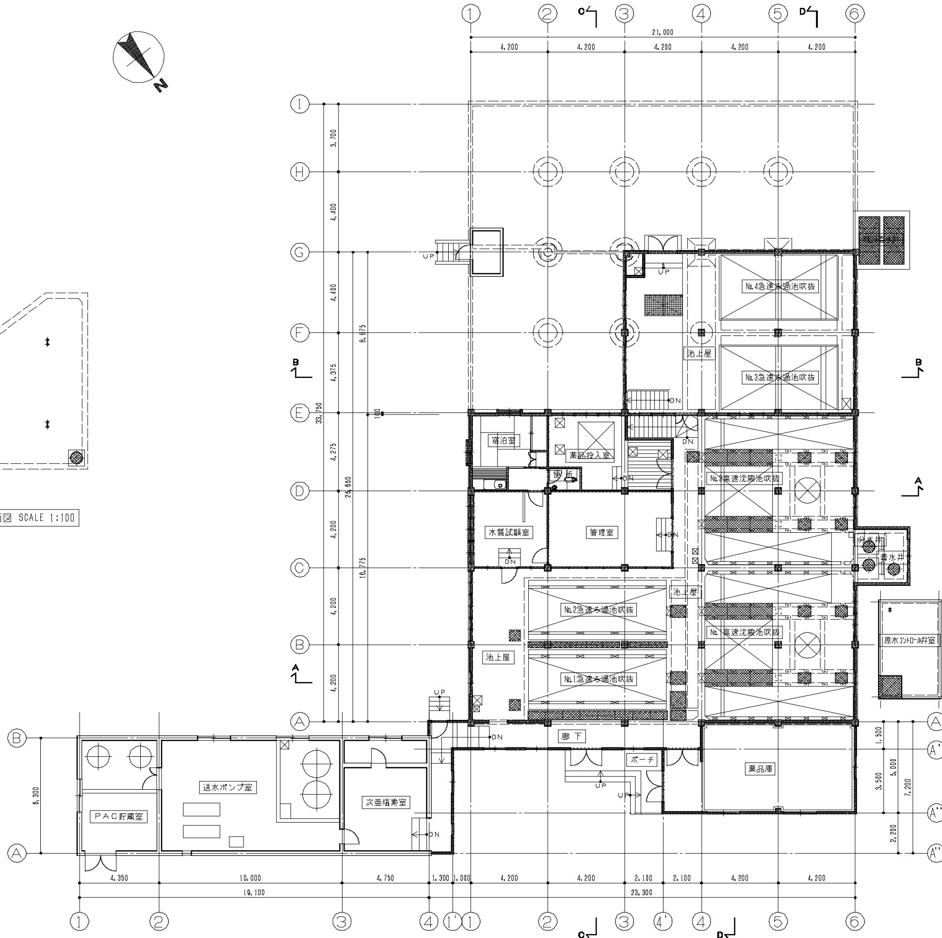
浄水場現況1階平面図 SCALE 1:100
