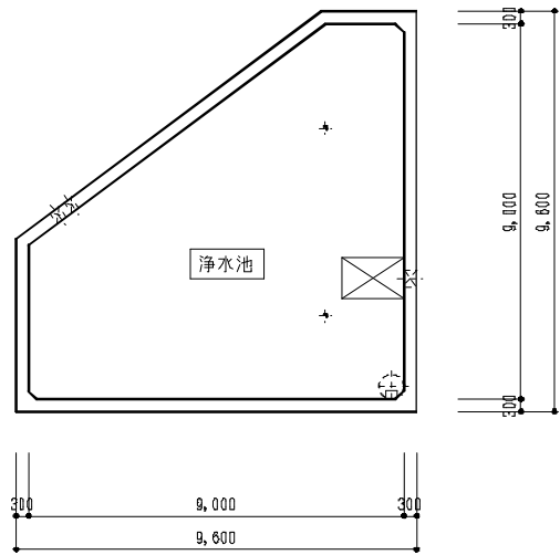
浄水池地階平面図 SCALE 1:100
