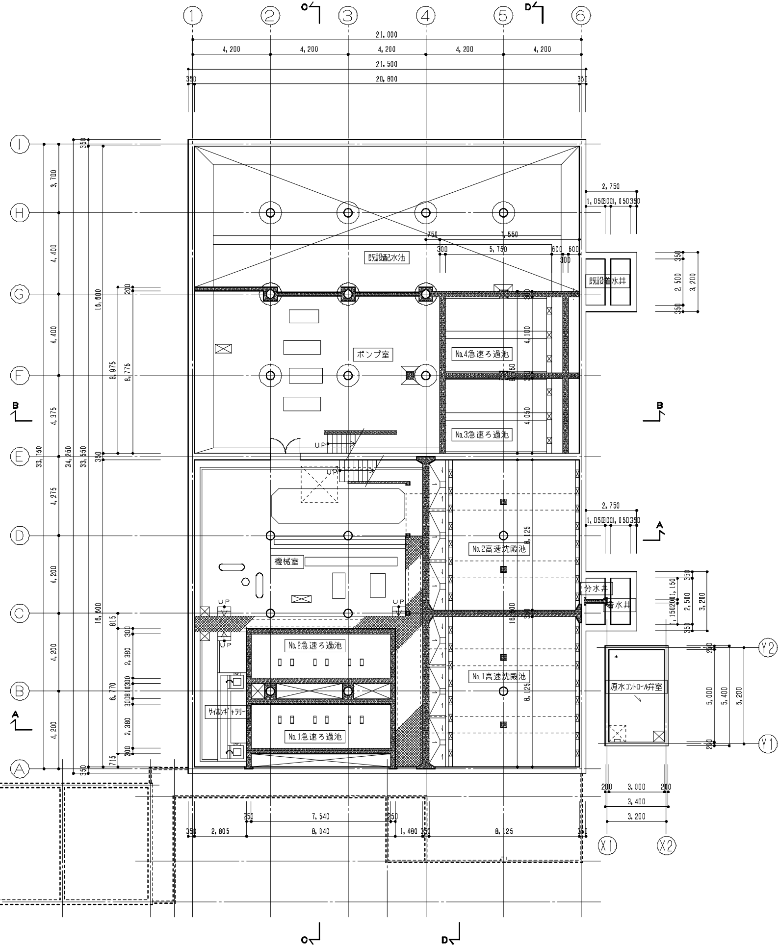
浄水場現況地階平面図 SCALE 1:100
